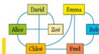
Doc. 2 Graphe des relations d'amitié
