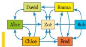
Doc. 3 Graphe des relations de suivi
